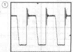
616 Vp-p 63.75kHz
