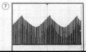
2Vp-p 100Hz
